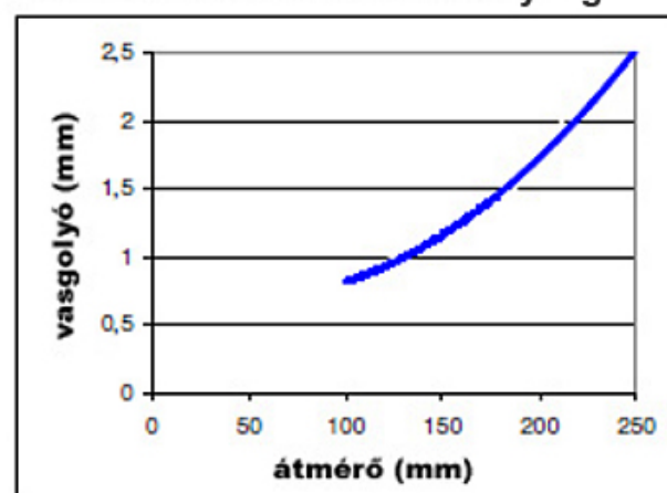
Fémérzékelés érzékenysége
